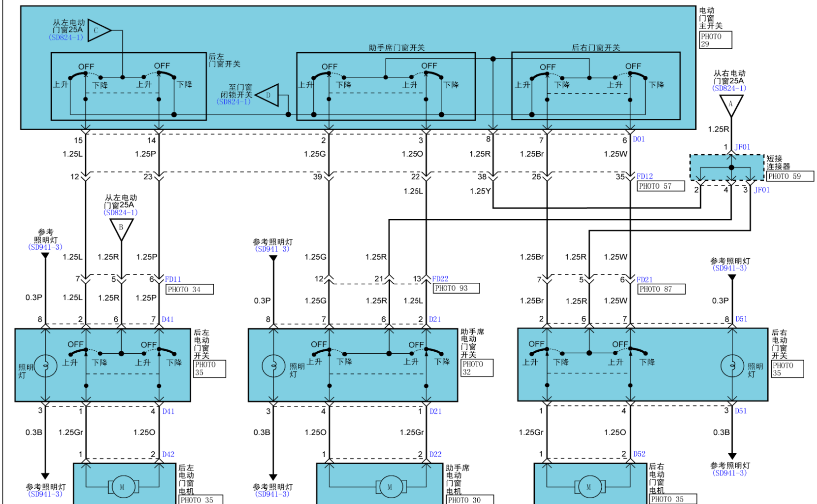
电动门窗 (2)
